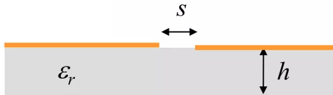
Slotline
